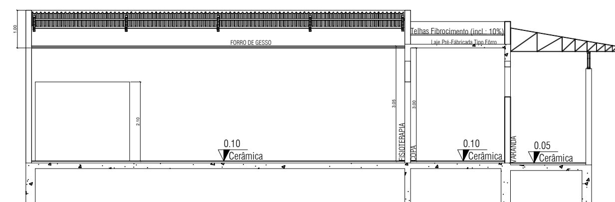
CORTE C-D Escala: 1/100
