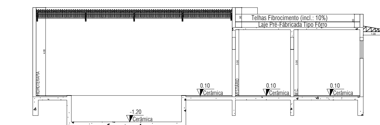
CORTE A-B Escala: 1/100
