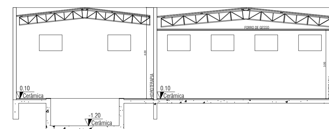
CORTE E-F Escala: 1/100
